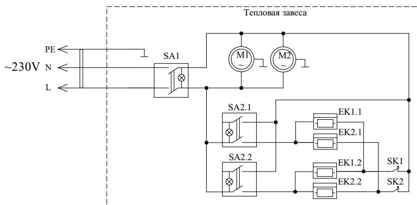
Рисунок 9. Принципиальная схема занавеси KVC-A08E3-11
