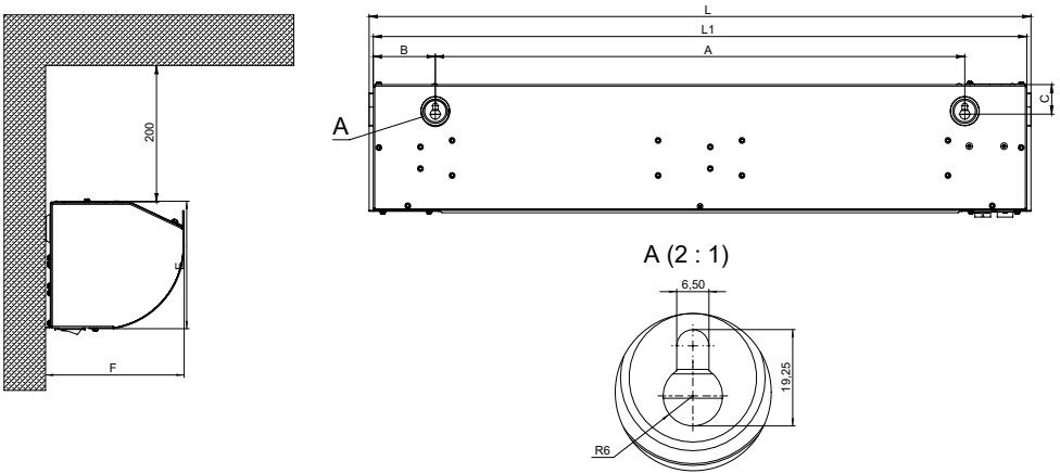
Рисунок 6. Габаритные и крепежные размеры
