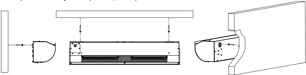
Рисунок 7. Схема крепления завесы горизонтально над проемом к стене с помощью отверстий на корпусе
