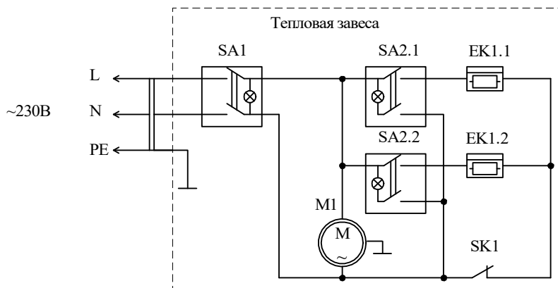
Рисунок 8. Принципиальная схема занавеси KVC-A06E3-11
