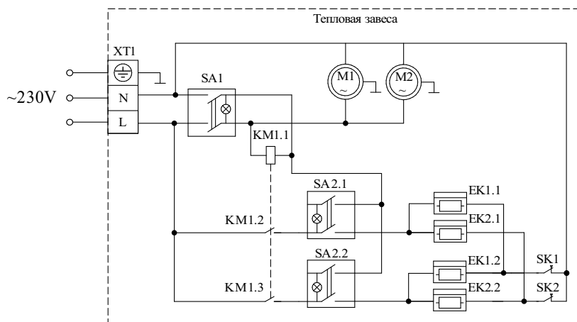
Рисунок 10. Принципиальная схема занесы KVC-A08E5-11
