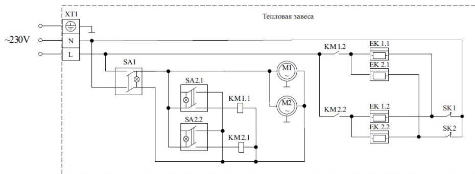
Рисунок 10. Принципиальная схема занесы KVC-A10E6-11
