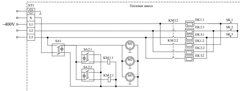
Рисунок 13. Принципиальная схема завесы KVC-A15E9-31
