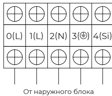
Клеммный терминал внутреннего блока
