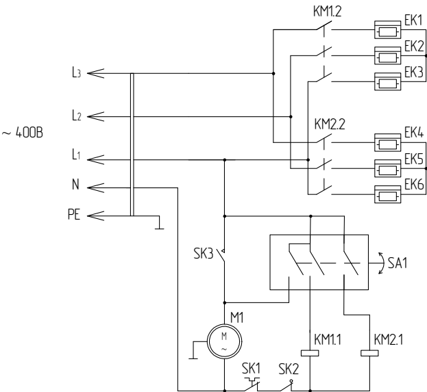
Схема коммутации переключателя
