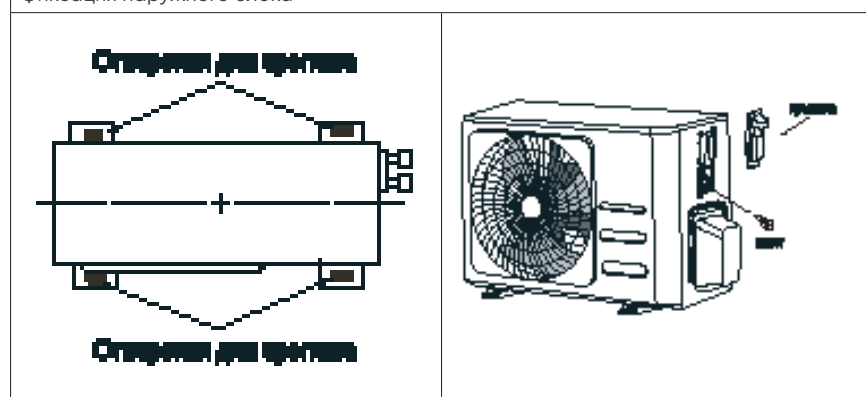
Фиксация наружного блока
